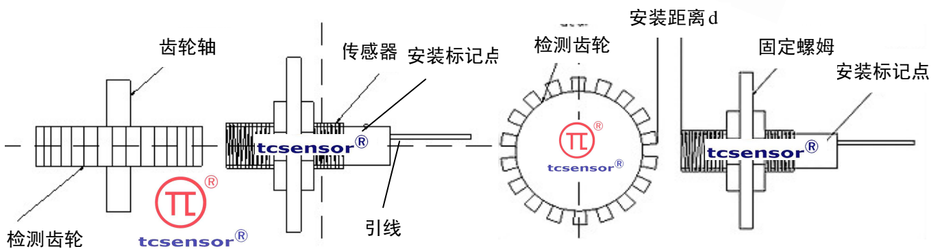
安装图示
